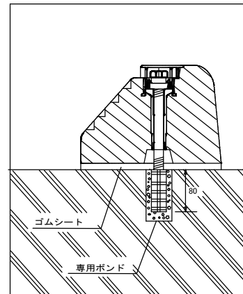
着脱式施工
